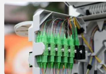
FTTx
